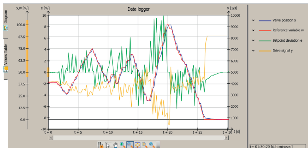
Fig. 2: Data logger
