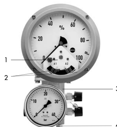
Fig. 2 · Media 5, Indicador 160 Ø con finales de carrera y bloque de válvulas con manómetro para presión de servicio acoplado
