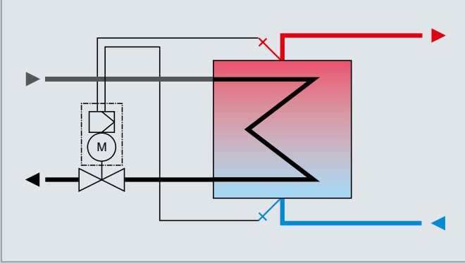
Tipik ısıtma uygulaması Dönüş hattı sıcaklık limitlemeli sıcaklık kontrolü
