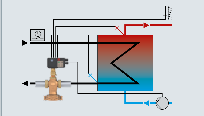
Régulation de chauffage en fonction des conditions climatiques de la température de départ avec limitation de la température de retour
