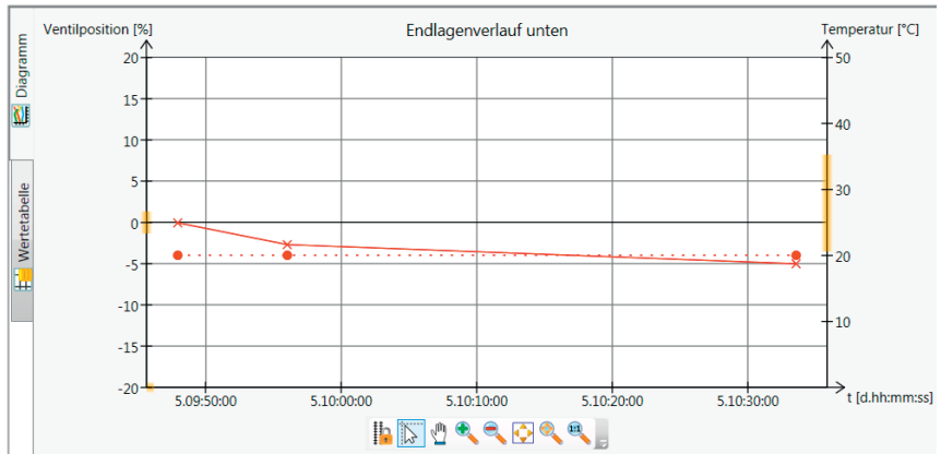
Bild 6: Unterer Endlagenverlauf
