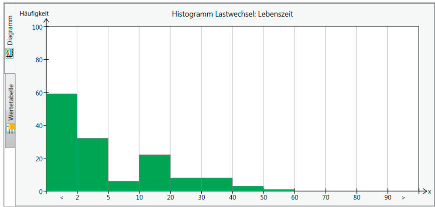
Bild 5: Histogramm Lastwechsel
