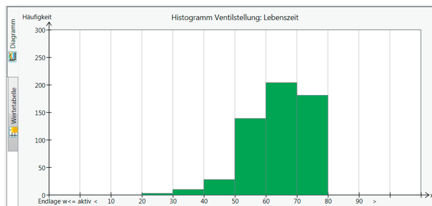
Bild 3: Histogramm Ventilstellung
